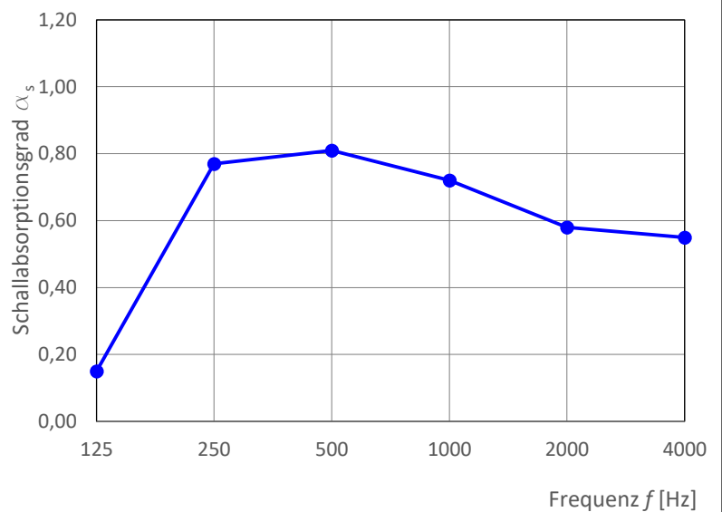
Schallabsorptionsgrad nach DIN EN ISO 354
